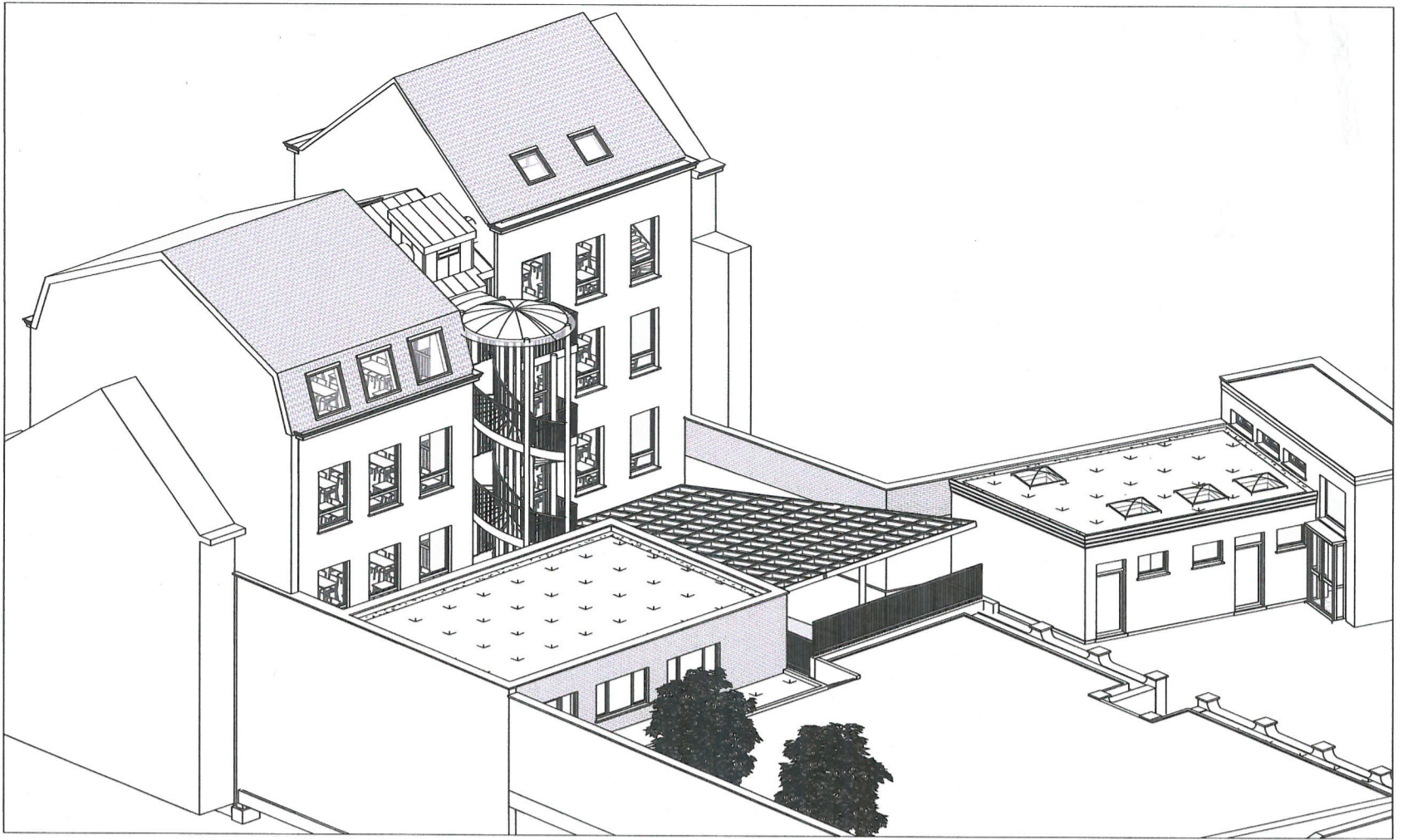
3D - FAÇADE ARRIÈRE - INTÉRIEUR DE L'INSTITUT
