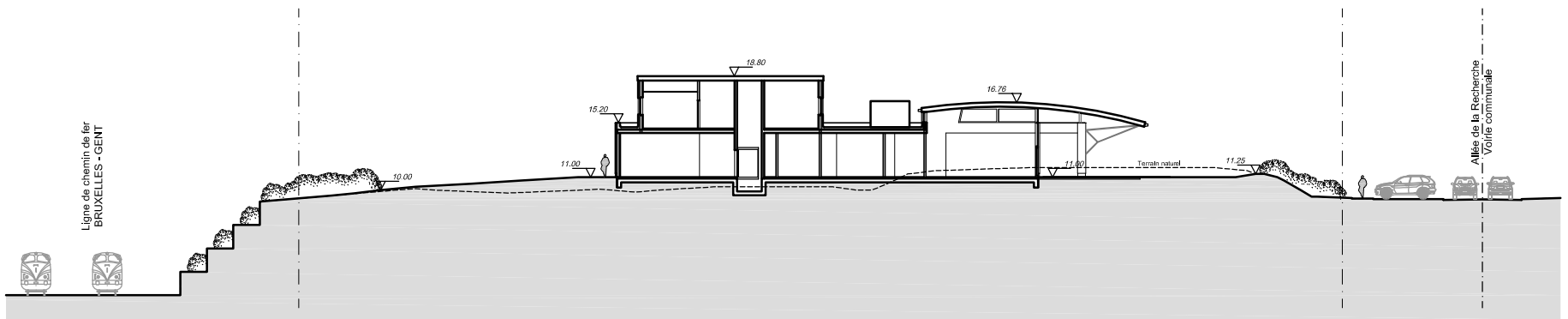
PROFIL D'IMPLANTATION BB 1/500
