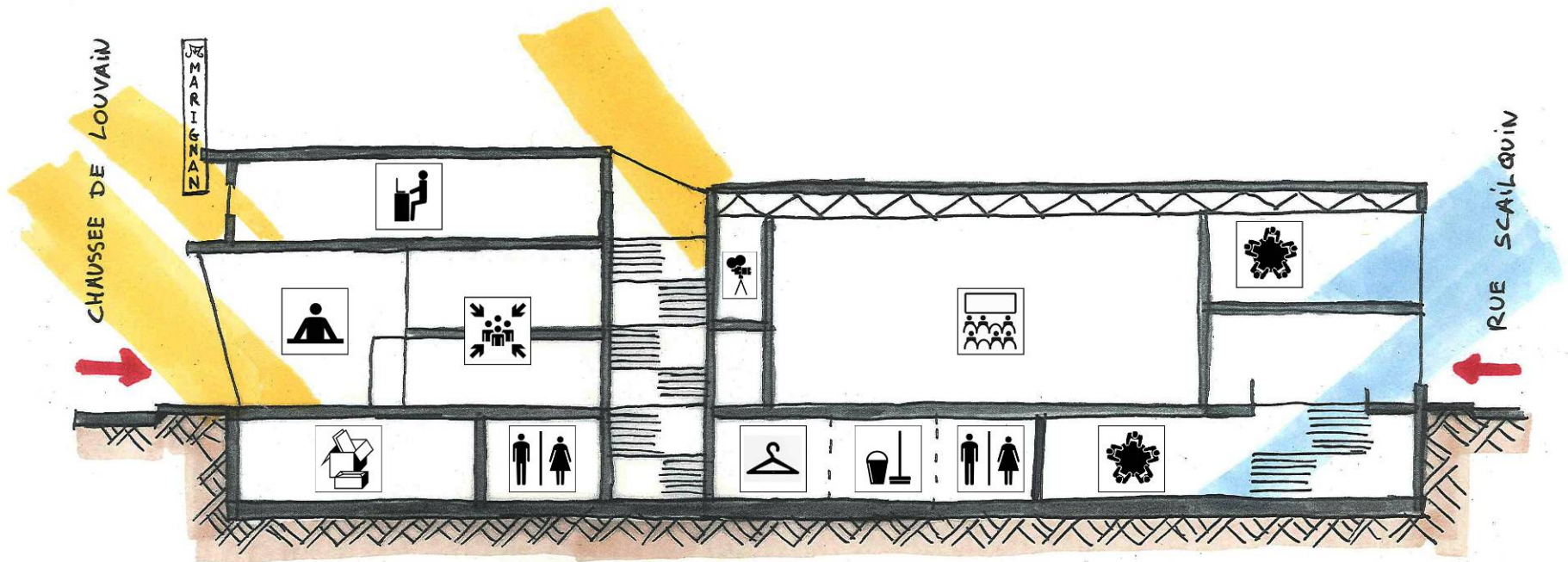
COUPE LONGITUDINALE
