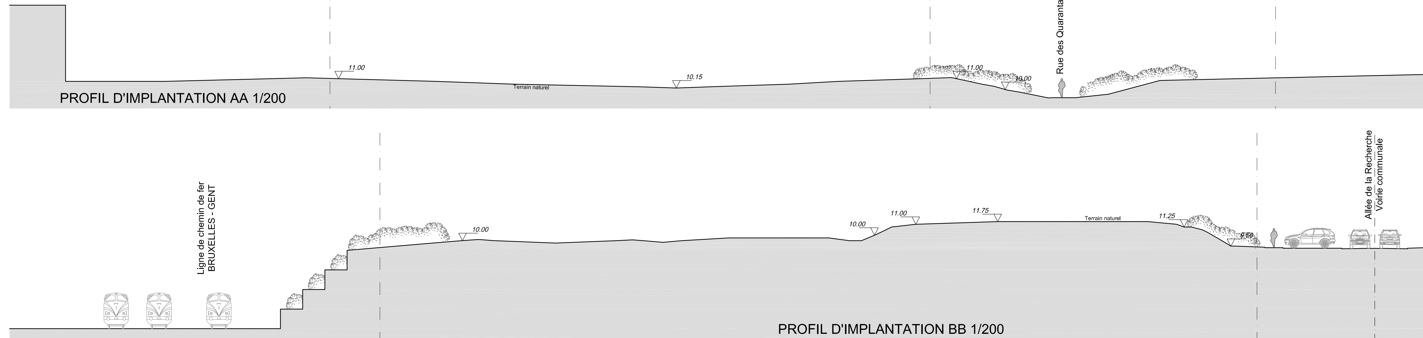
PROFIL D'IMPLANTATION BB 1/200
